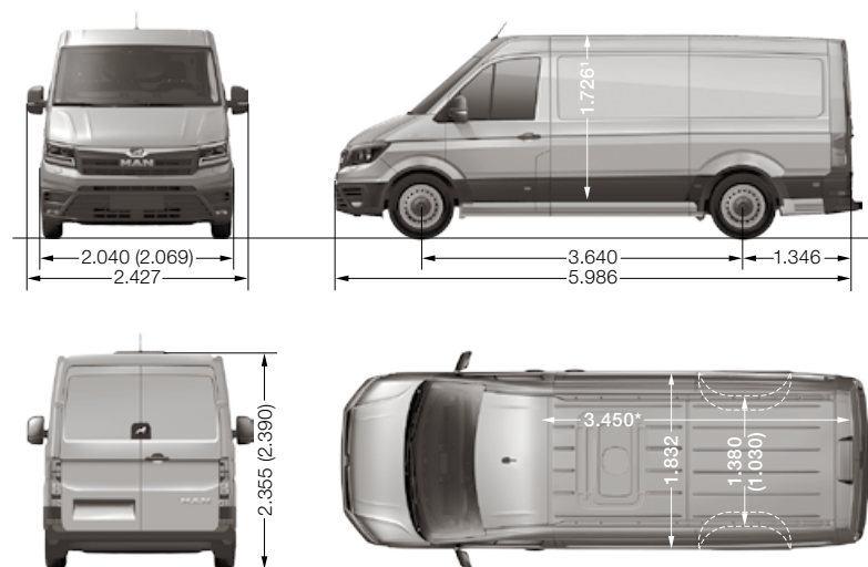
MAN TGE Furgone Standard con Tetto normale
