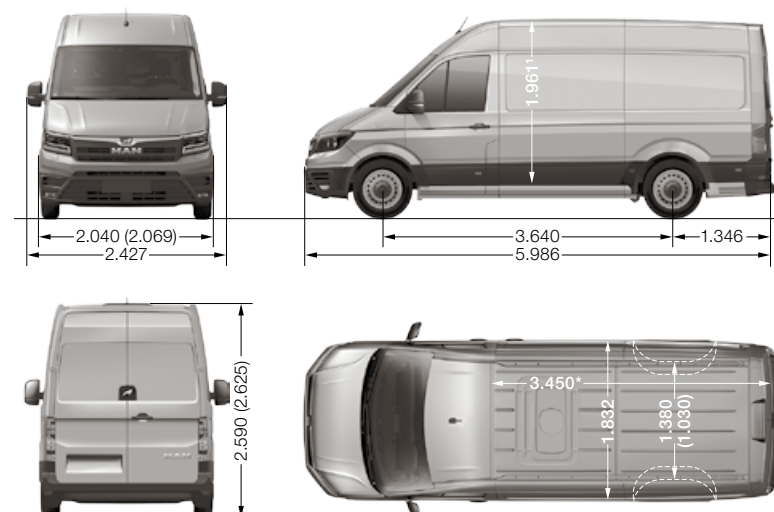
MAN TGE Furgone Standard con Tetto alto
