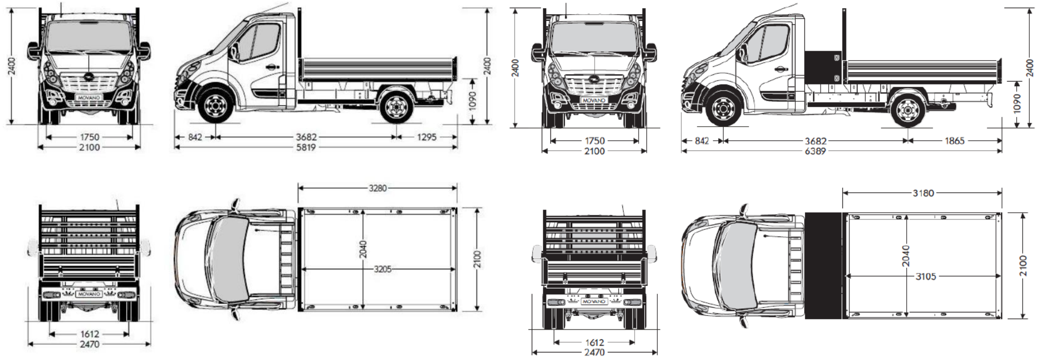
Ribaltabile - L2 - T. Posteriore Gemellato
