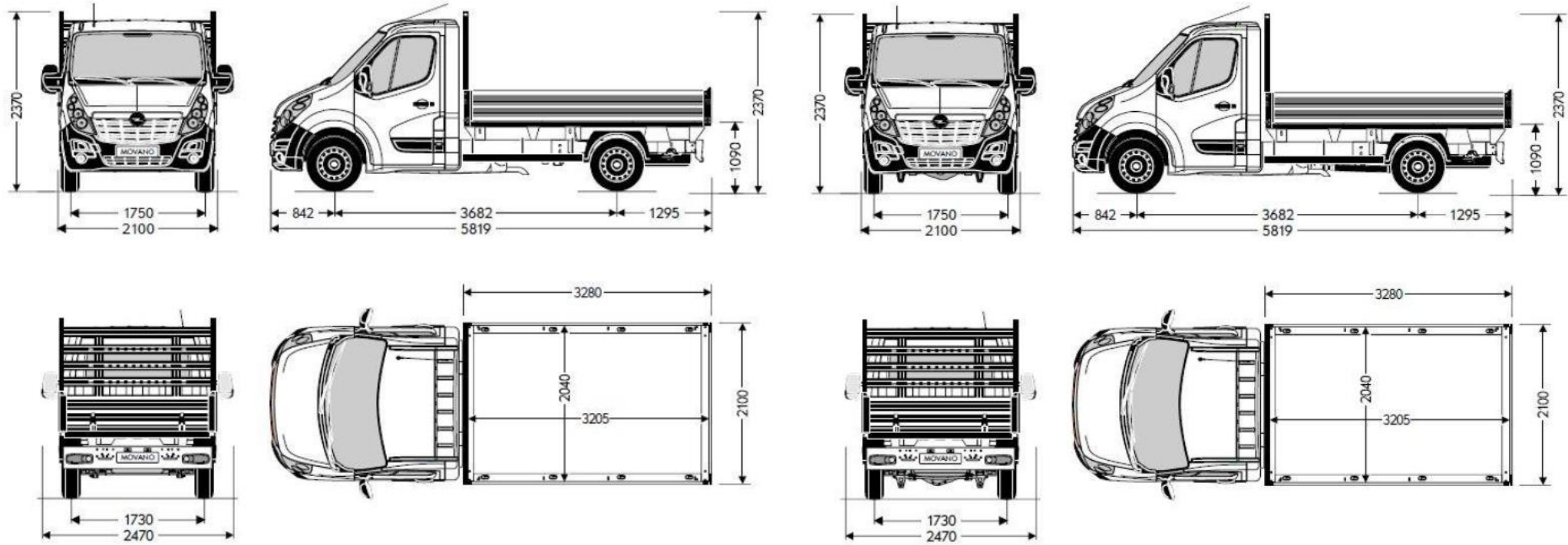
Ribaltabile - L2 - T. Anteriore
