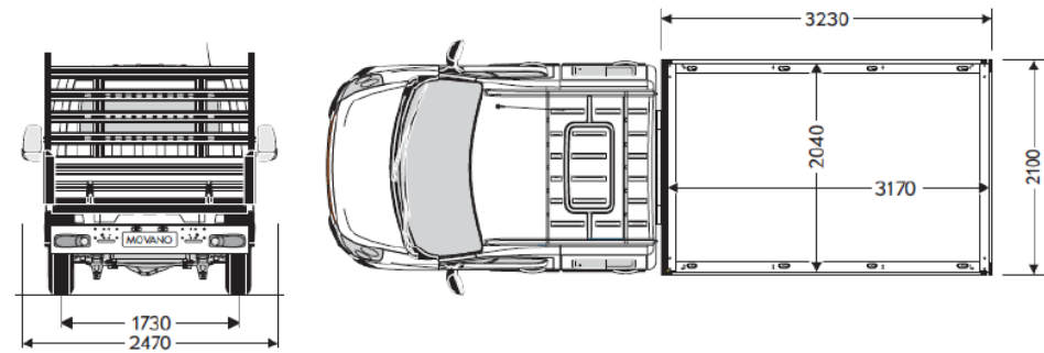
Doppia Cabina - Fisso - L3 - T. Posteriore
