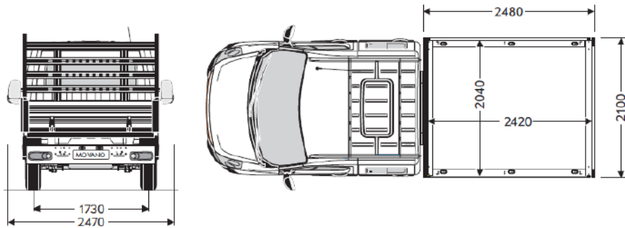
Doppia Cabina - Fisso - L2 - T. Anteriore
