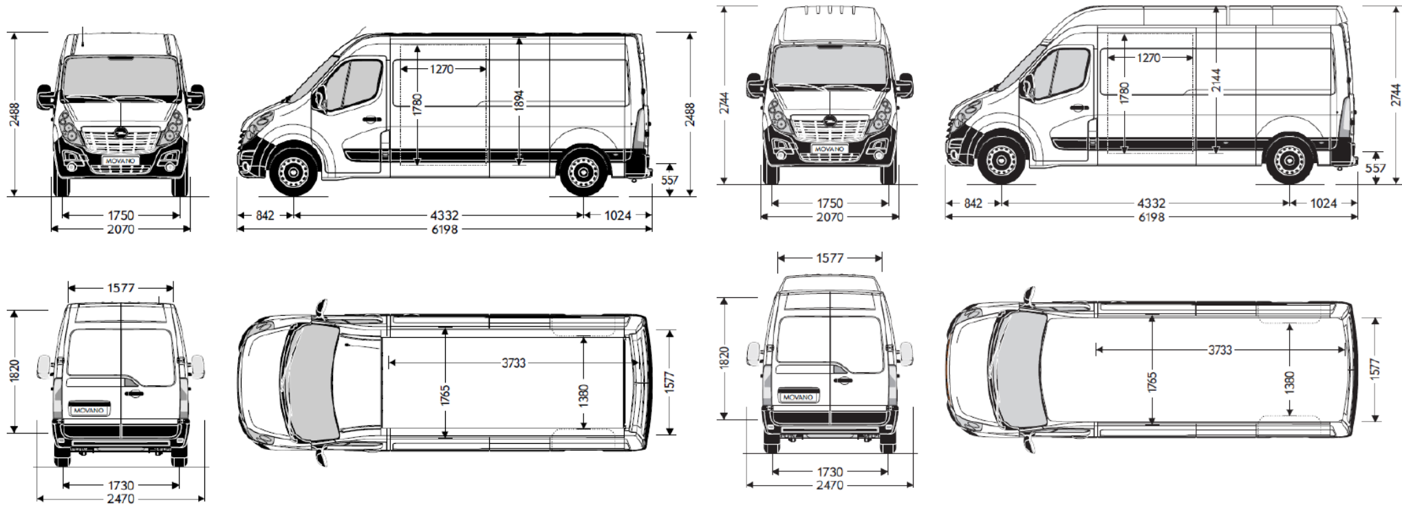
L3H2 – T. Anteriore
