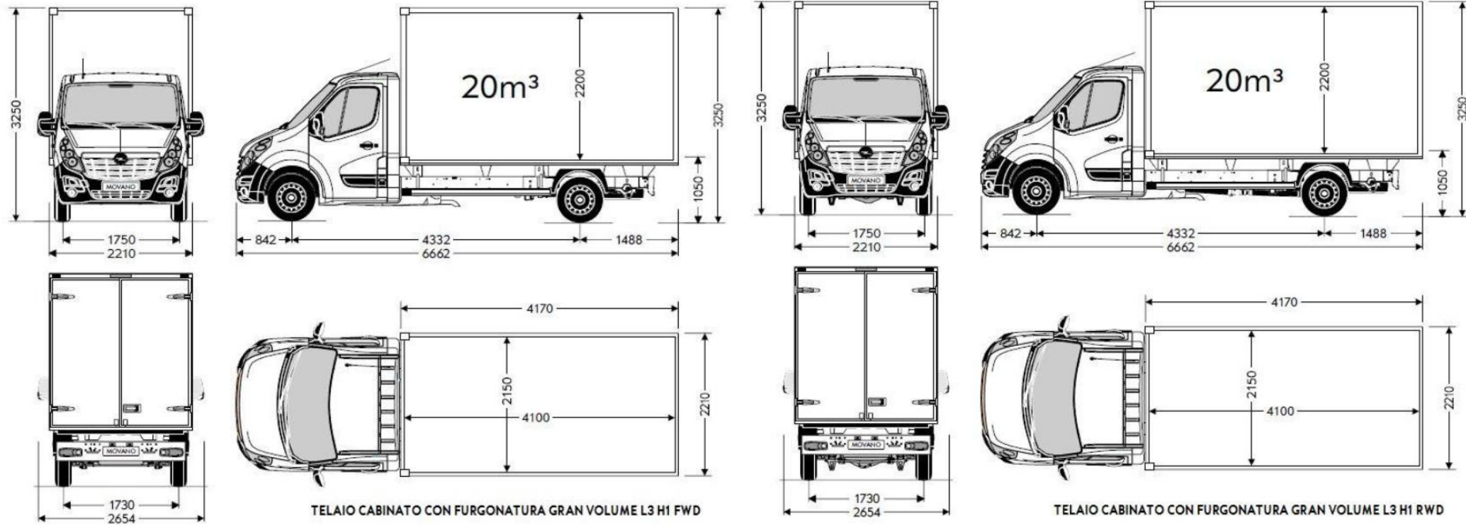
Furgonato - L3 - T. Anteriore
