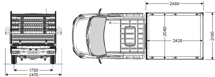
Doppia Cabina - Fisso - L2 - T. Posteriore
